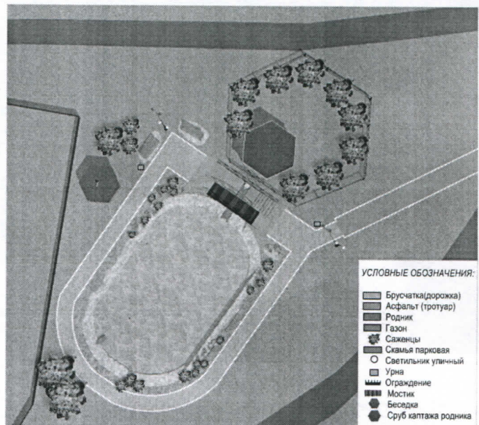
ГЕНЕРАЛЬНЫЙ ПЛАН БЛАГОУСТРОЙСТВА
